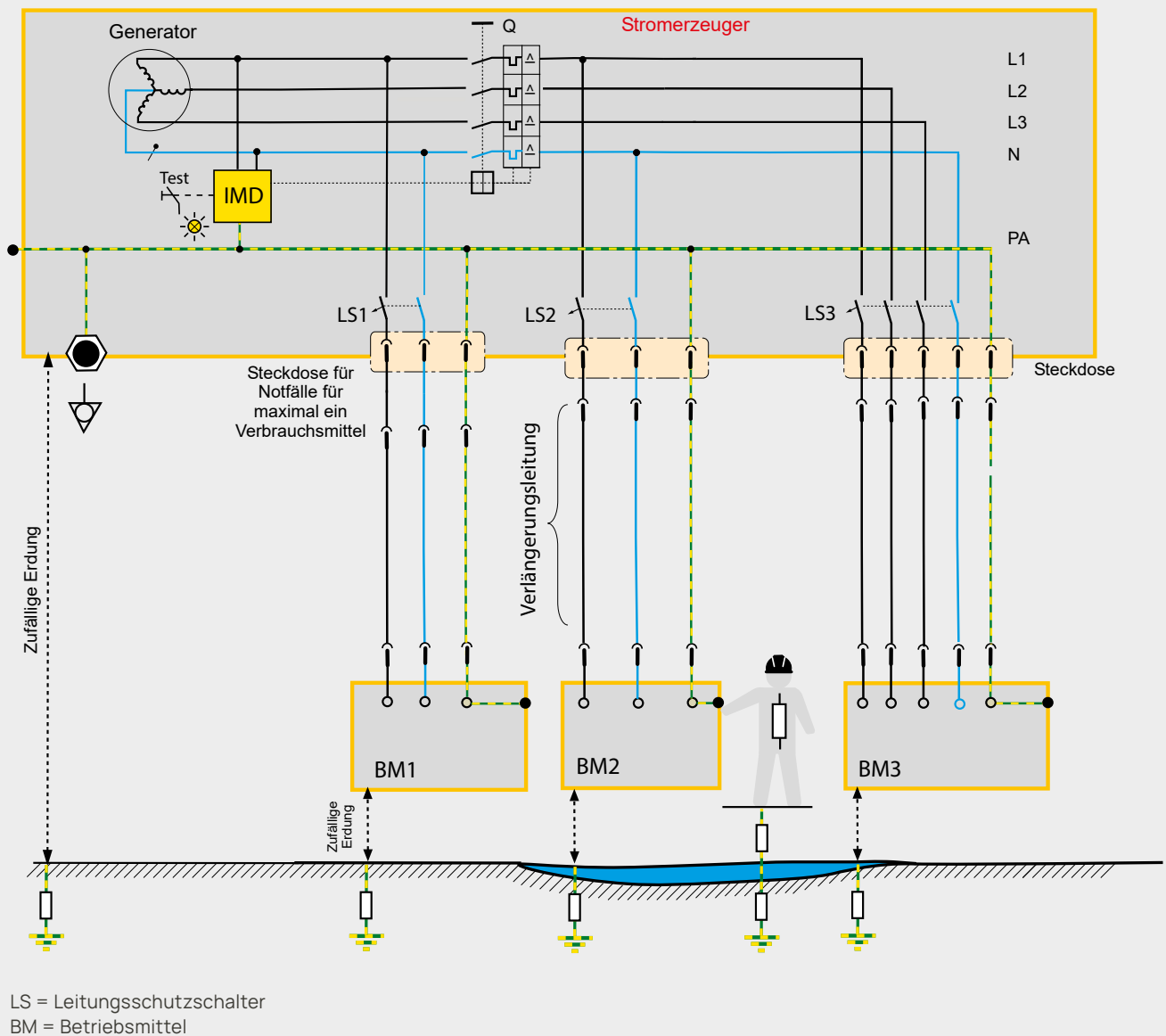
Schutztrennung mit Isolationsüberwachungseinrichtung (IMD) und automatischer Abschaltung
