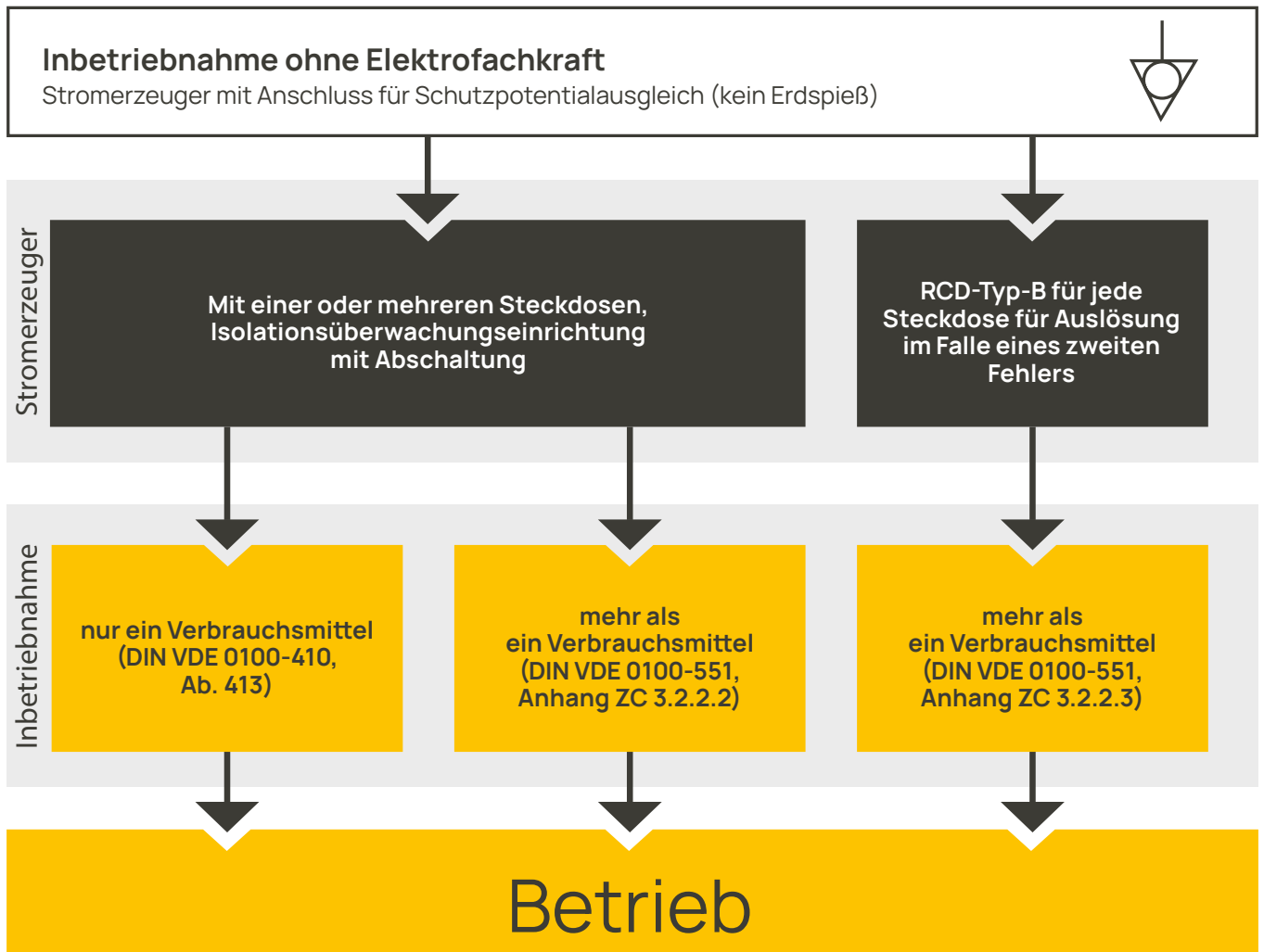
Bild 1: Möglichkeiten für den sicheren und ordnungsgemäßen Betrieb von mobilen Stromerzeugern
